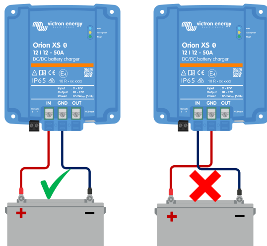
Beispiel für richtige und falsche (vertauschte) Batteriepolartät:
